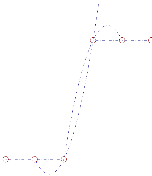
Abbildung 17: Entstehung von Oszillationen
