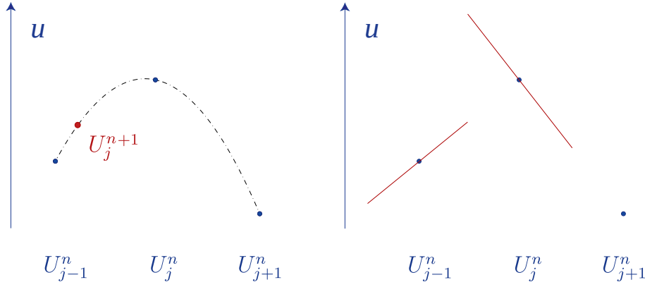
Abbildung 15: Zwei Sichtweisen für das Lax-Wendroff-Verfahren
