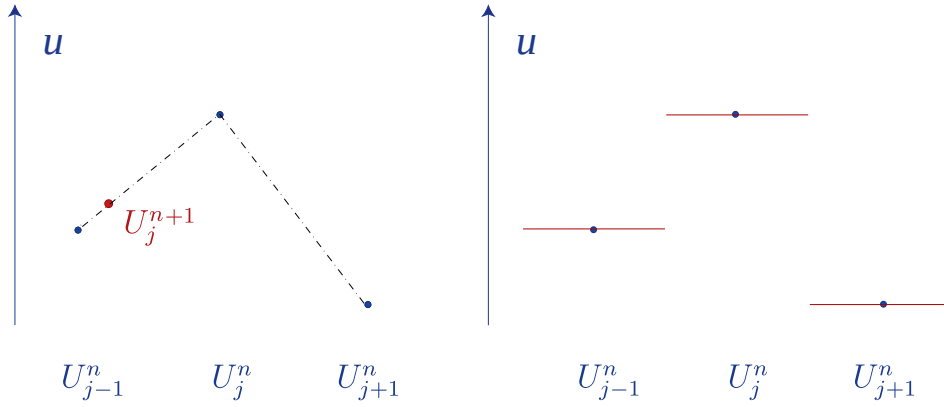
Abbildung 14: Zwei Sichtweisen für das Upwind-Verfahren
