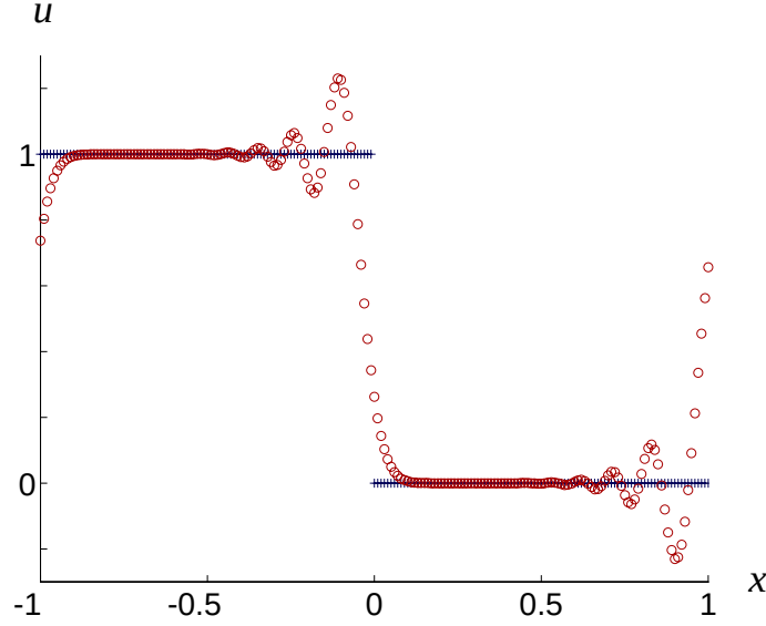
Abbildung 13: Lax-Wendroff Dispersion an unstetiger Lösung
