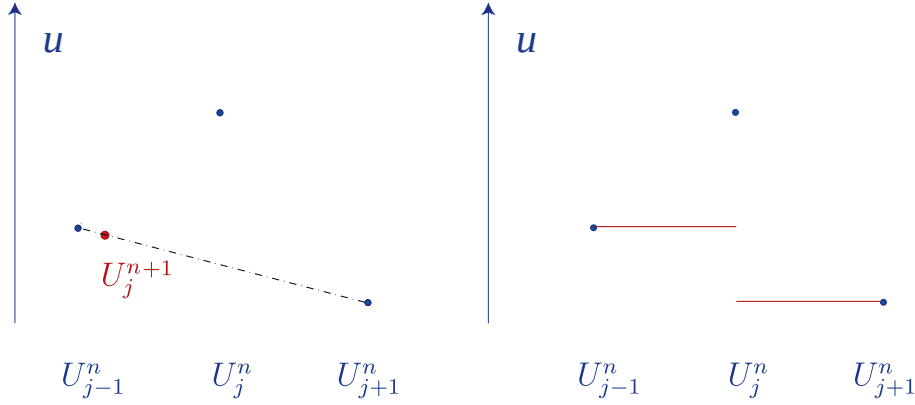
Abbildung 16: Zwei Sichtweisen für das Lax-Friedrichs-Verfahren
