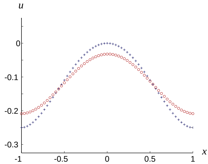
Abbildung 8: Lax-Friedrichs Diffusion an glatter Lösung
