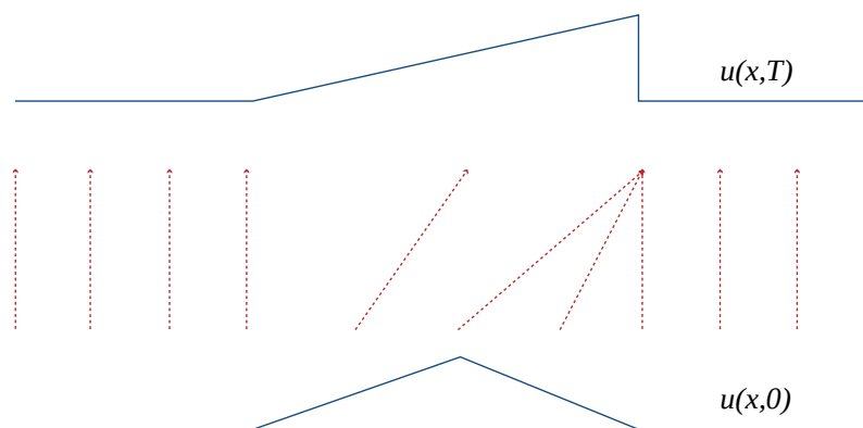
Abbildung 5: Schockbildung bei Burgers' Gleichung
