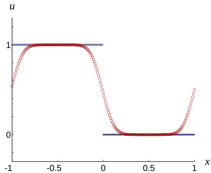
Abbildung 11: Upwind Diffusion an unstetiger Lösung
