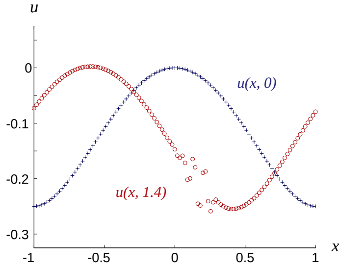
Abbildung 7: Instabilität bei Verletzung der CFL-Bedingung
