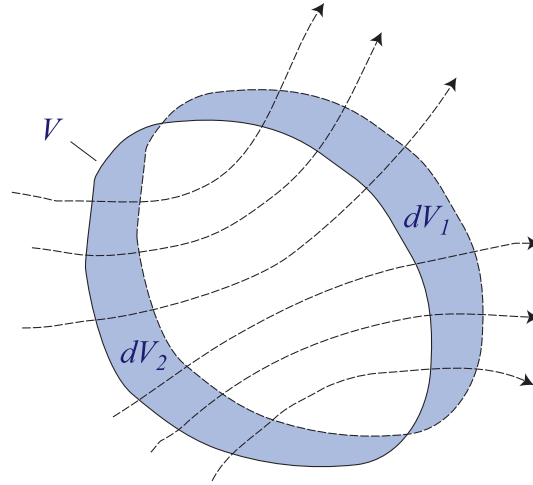
Abbildung 2: Massenerhaltung
