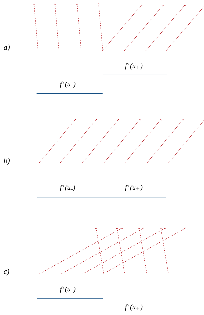
Abbildung 6: Schockausbreitung bei stückw. konst. Anfangswerten
