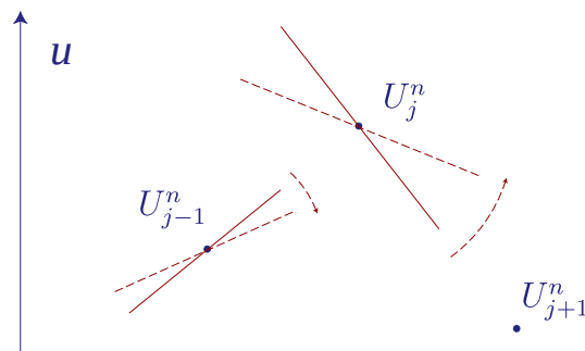
Abbildung 18: Slope limiter
