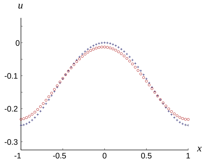
Abbildung 10: Upwind Diffusion an glatter Lösung
