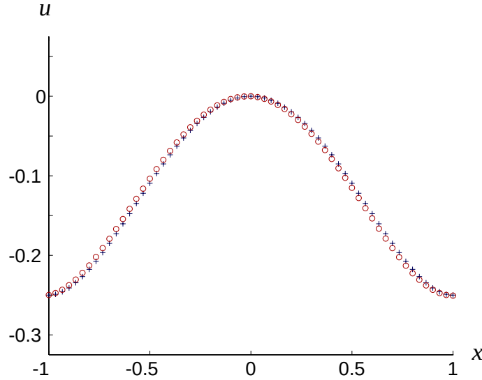
Abbildung 12: Lax-Wendroff Dispersion an glatter Lösung
