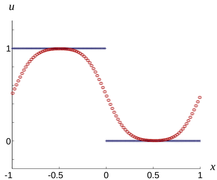
Abbildung 9: Lax-Friedrichs Diffusion an unstetiger Lösung
